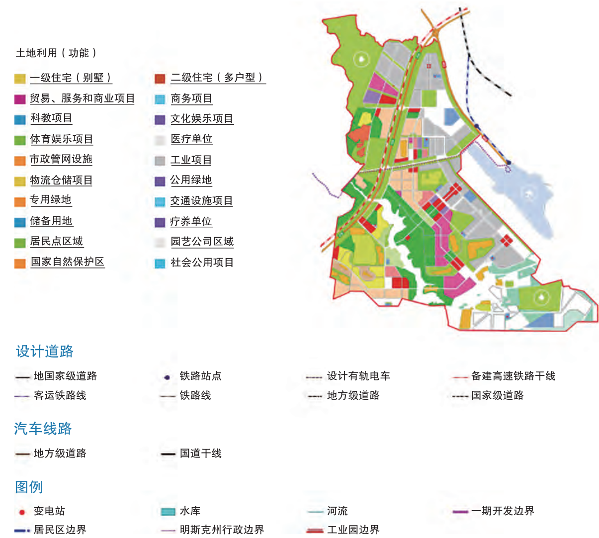
图 3-4 中白工业园规划图
